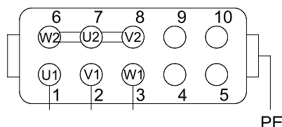
Stern-Schaltung (Y)
