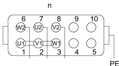
YY-Schaltung
