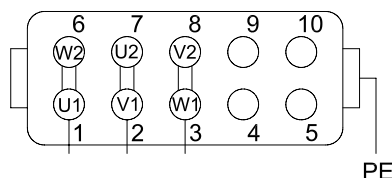
Dreieck-Schaltung (Δ)
