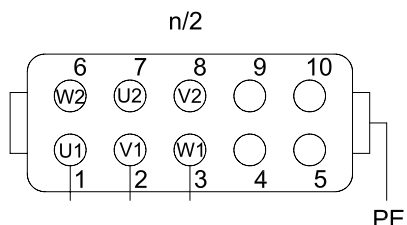
Y-Schaltung
